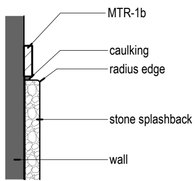
3 Stone Splashback & Batten 1 : 5
