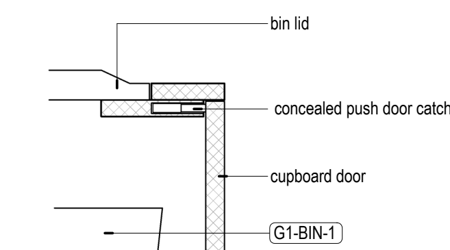
18 Bin / Cpd 1 : 5
