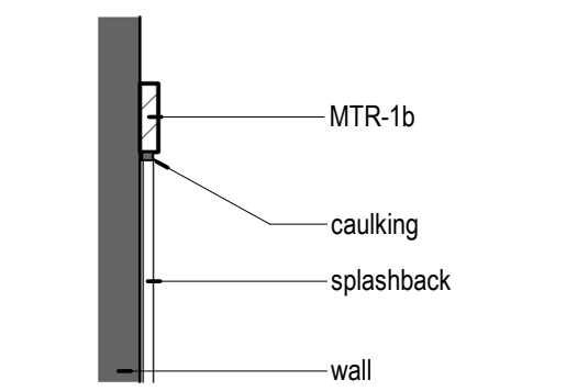
1 Splashback & Batten 1 : 5
