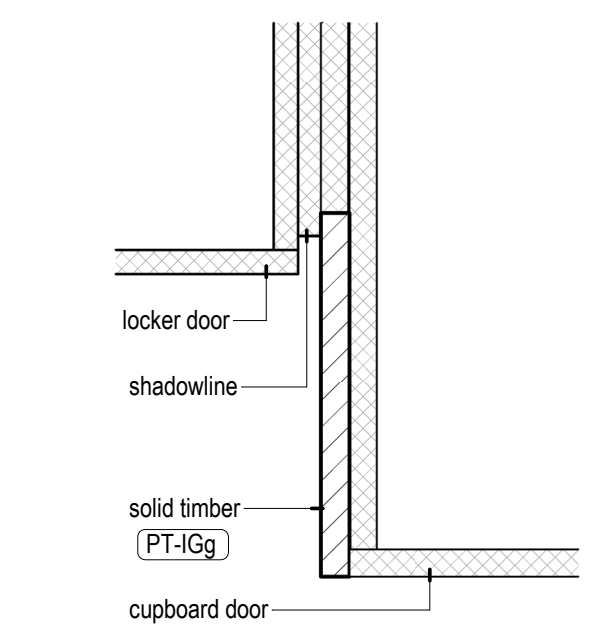
27 JO-St-2 - Door 1 : 5 Plan Detail
