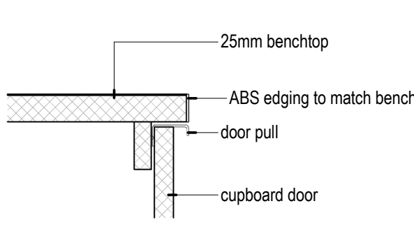
11 Bench / Cpd 1 : 5
