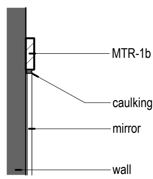
4 Mirror & Batten 1 : 5
