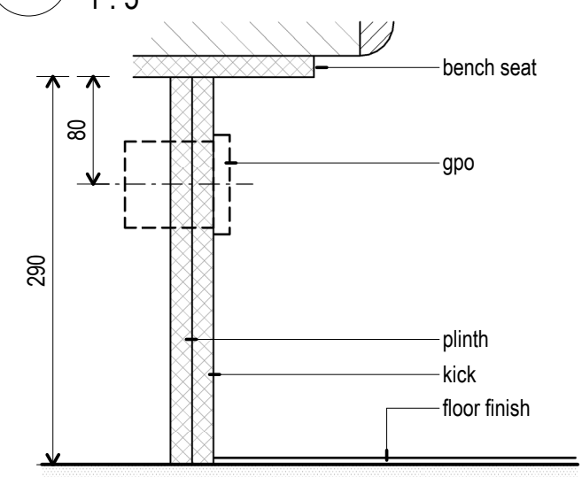
23 JO-SE-2 Plinth 1 : 5
