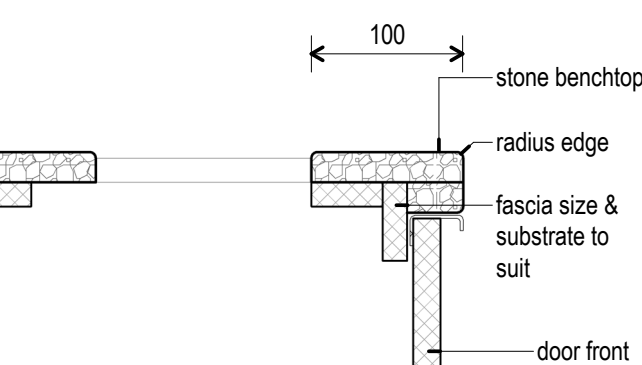
11 Bench / Cpd 1 : 5
